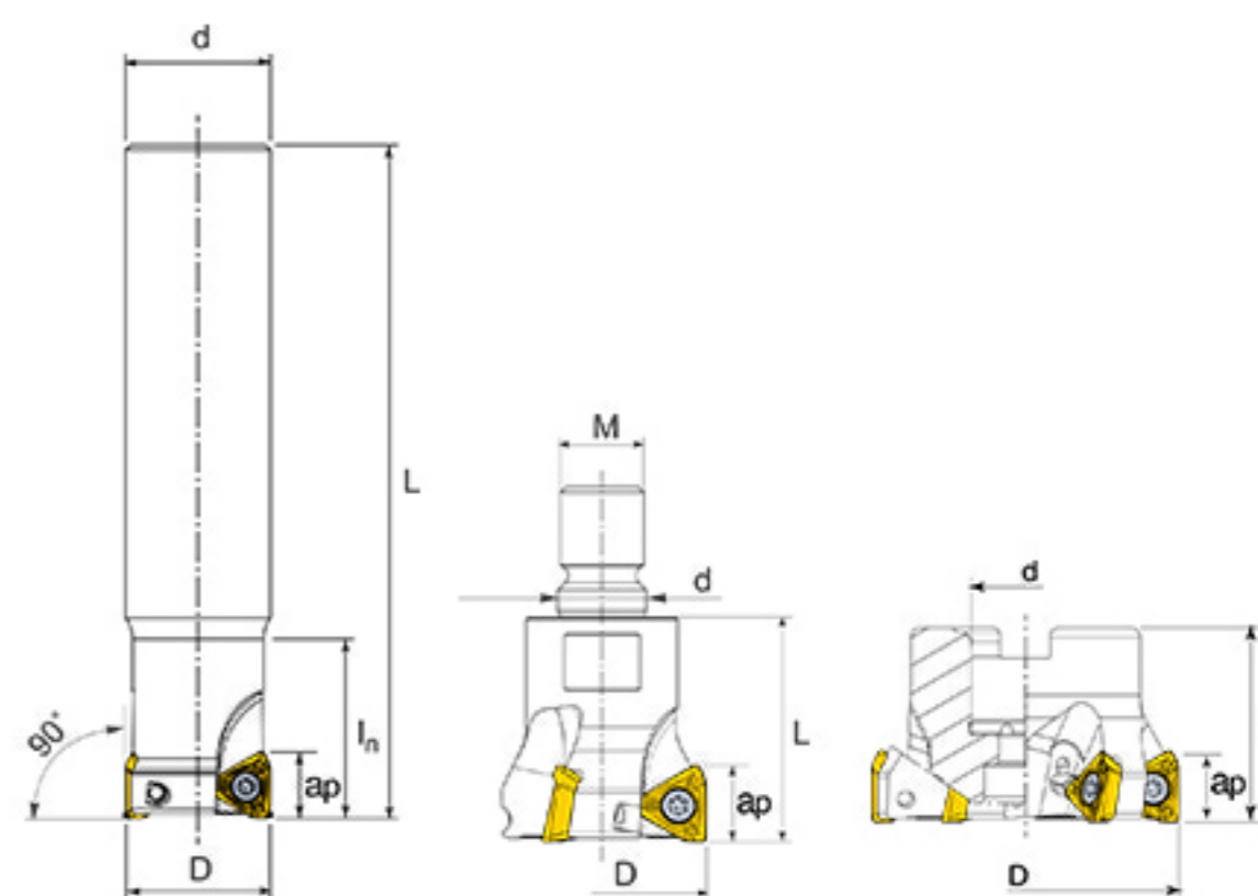
ЦИЛИНДРИЧЕСКИЙ ХВОСТОВИК
